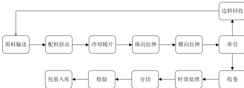
图：新型薄膜材料主要工艺流程
