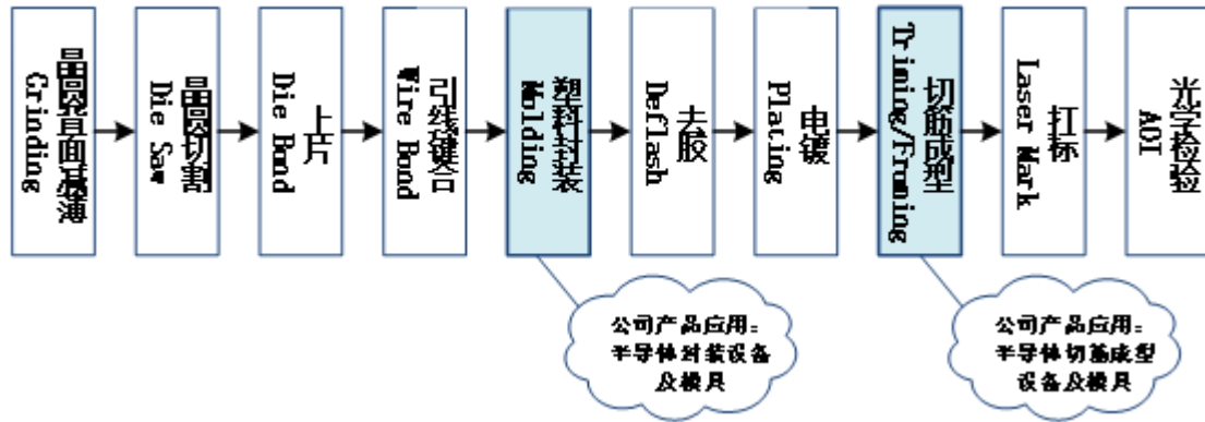
芯片封装工艺流程
