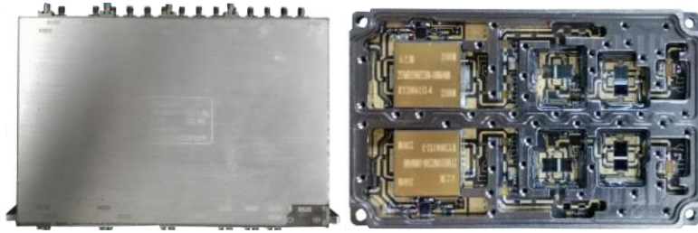
图：公司变频组件系列产品
