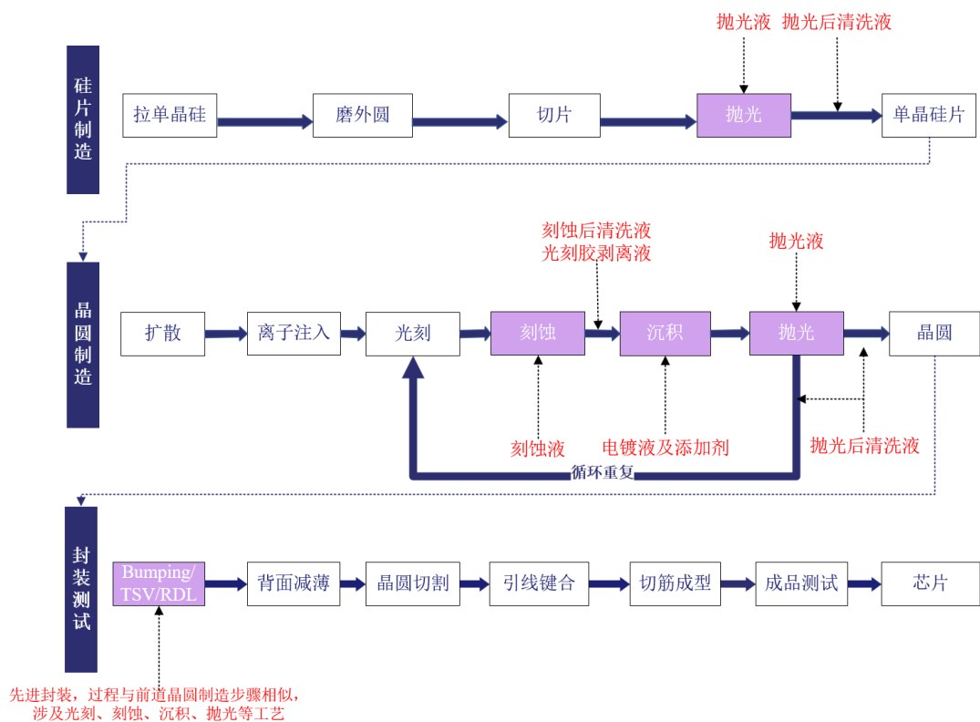
公司主要产品在芯片制造及先进封装领域的关键循环重复工艺中多次应用
