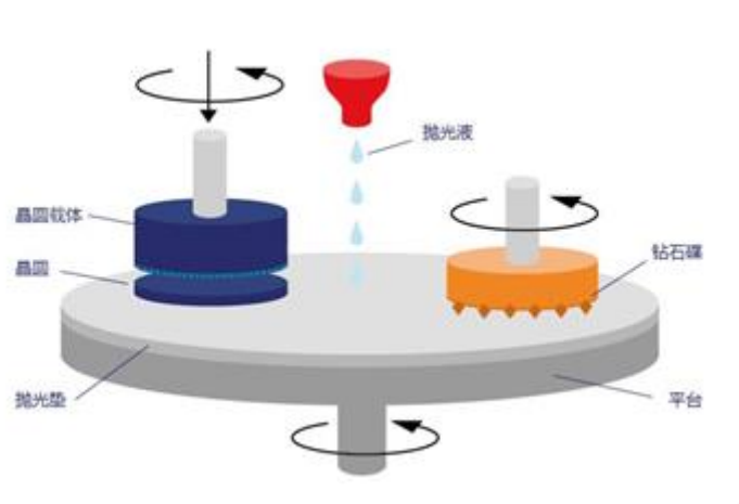
CMP 工艺原理图
