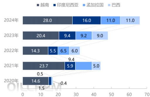
2020-2024 年度中国聚丙烯出口量对比图 --按目的地 (万吨)
